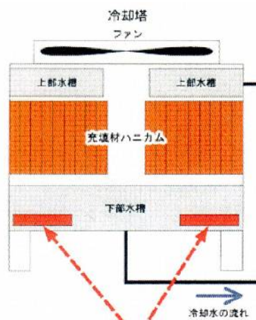
設置例
